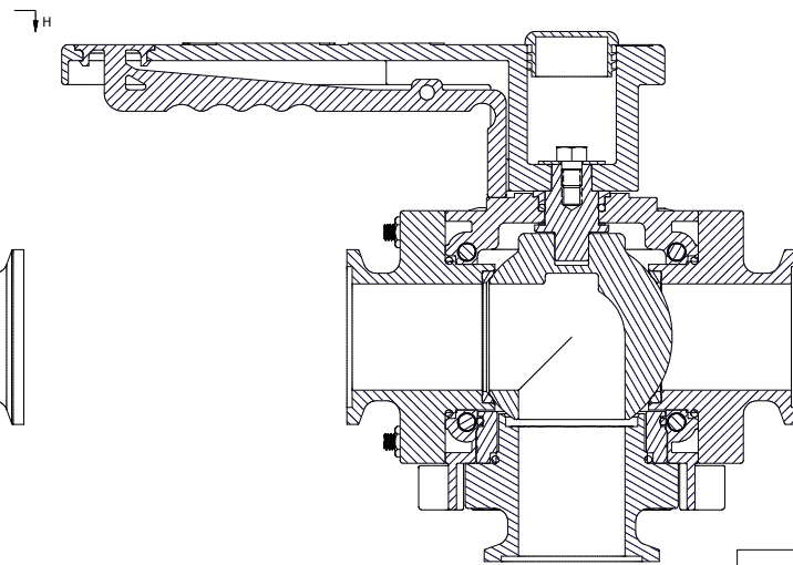
SECTION G-G SCALE 1 : 1
